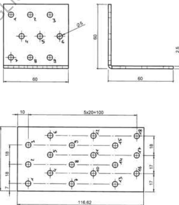
Abb. B. 6 Abmessungen des Winkelverbinders 631 640 25
