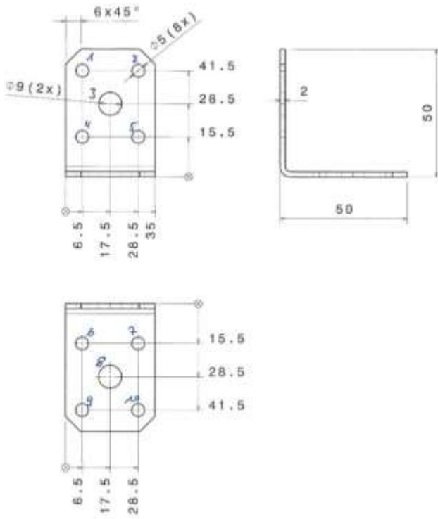
Abb. B. 77 Abmessungen des Winkelverbinders 641 553 20
