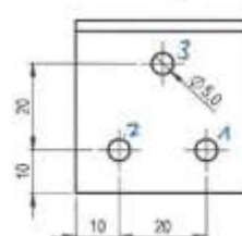
Abb. B. 64 Abmessungen des Winkelverbinders 631 444 25
