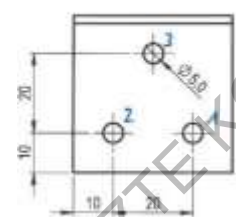
Abb. B. 63 Abmessungen des Winkelverbinders 631 444 20
